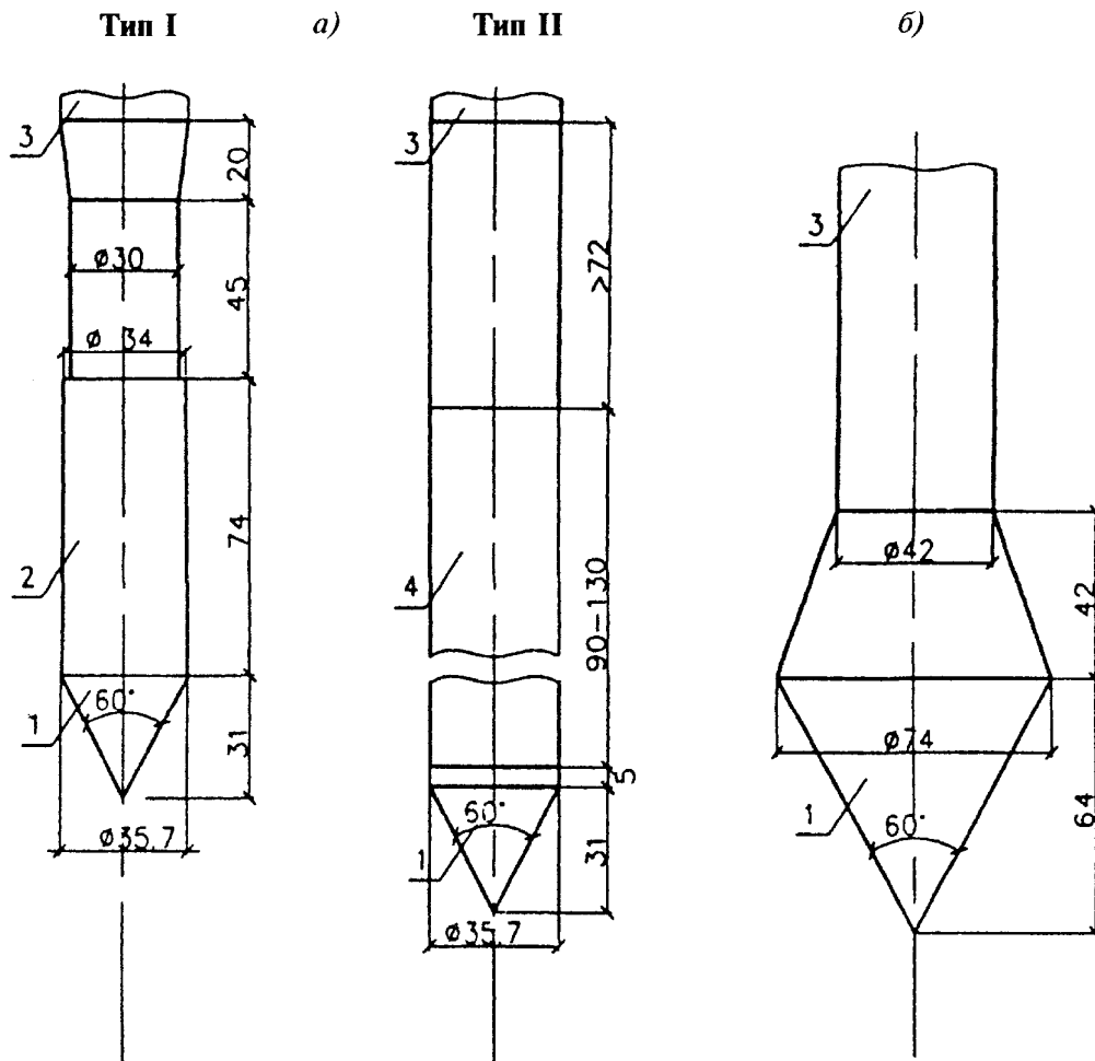
a — для статического зондирования; б — для динамического зондирования (ударного); 1 — конус; 2 — кожух; 3 — штанга; 4 — муфта трения
